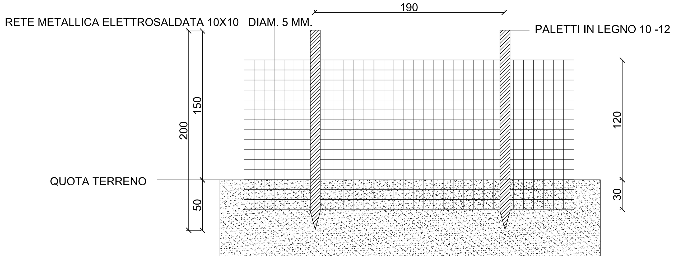
PARTICOLARE RECINZIONE
