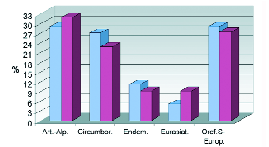
Fig. 2 - Spettri corologici dei due popolamenti centro-appenninici rilevati.
