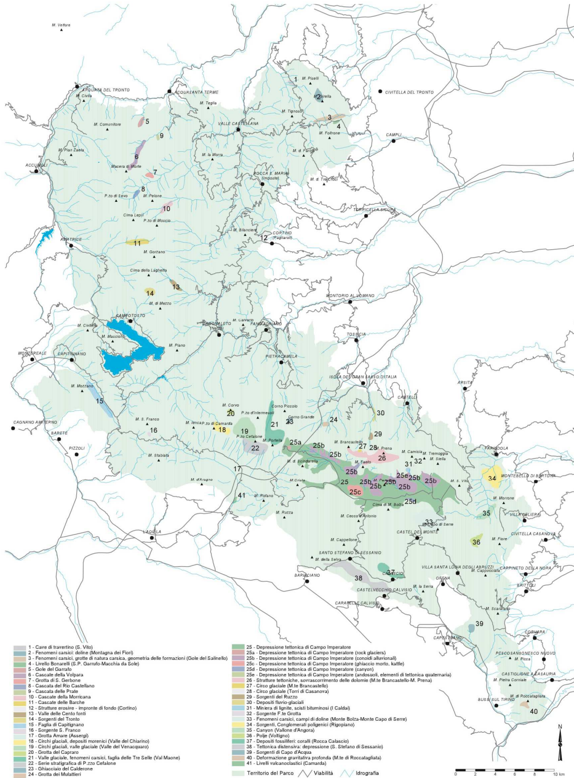
TAV. 2 - EMERGENZE GEOLOGICHE
