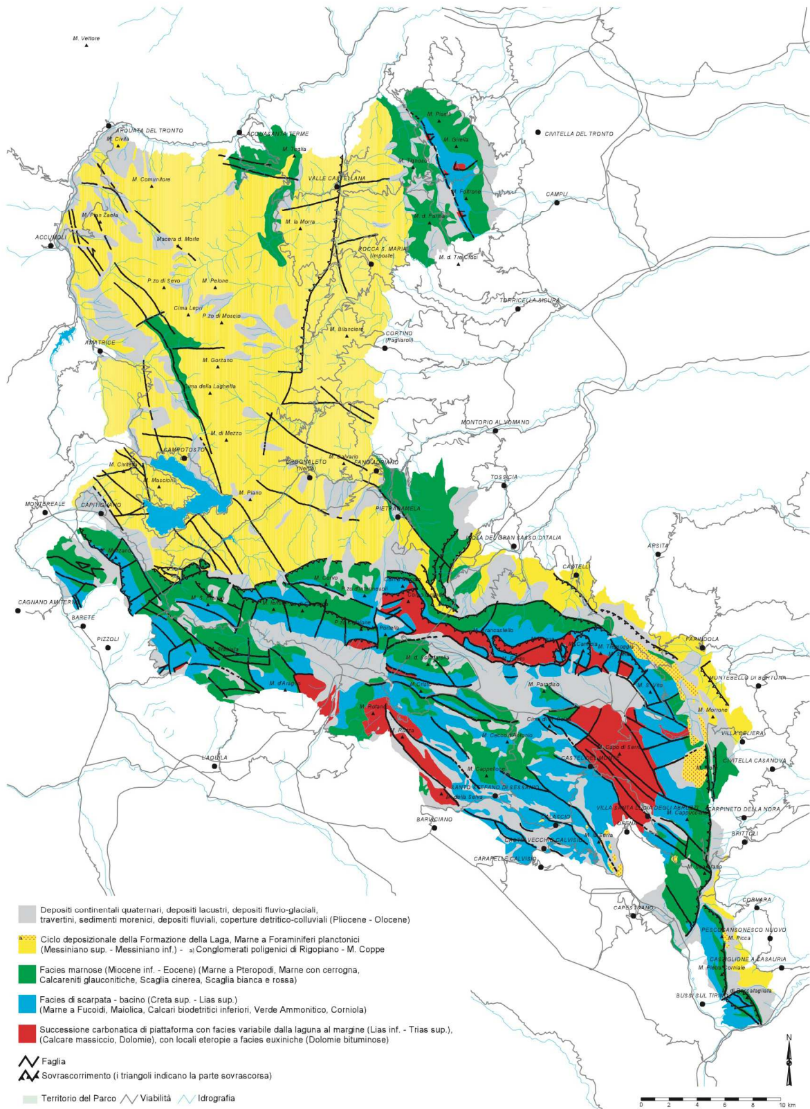
TAV. 1 - GEOLITOLOGIA
